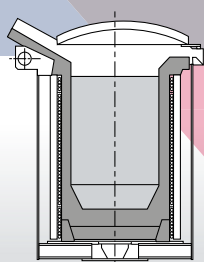
Coreless induction furnaces \ Horno inducción crisol
